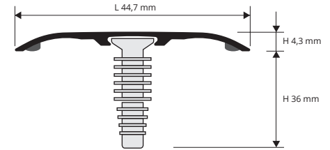
PMPFX... 42090AS / 42A escala 1:1
