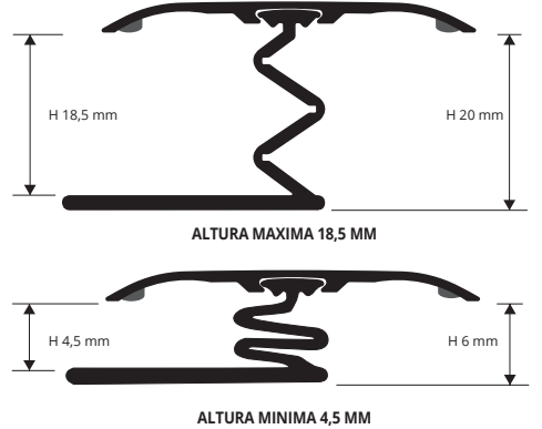
PMPFX... 42090AS / 42A + PMFIXBSAN 23 escala 1:1
