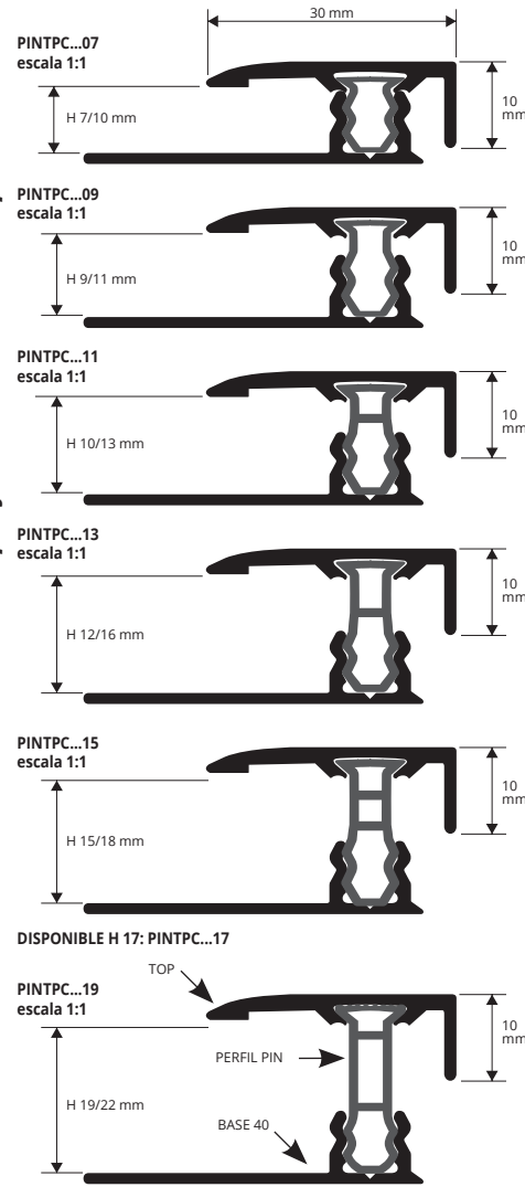
TOP ALU.+PERFIL PIN+BASE 40 ALU. AGUJERADA (6 acabados aluminio anodizado, 3 solo bajo pedido) thermo empaquetado - Unidades de 2,7 M de largo paq. de 20 UDS - 54 M (PIN 11, 15, 17 - 40,5 M) (PIN 19 - 27 M)
