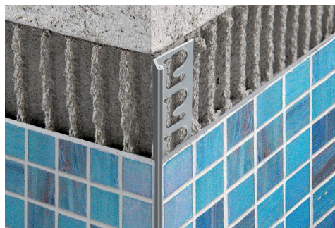
ACERO INOX AISI 304/1.4301-V2A BRILLO con película protectora Unidades de 2,7 M de largo - Paq. de 40 UD - 108 ml
